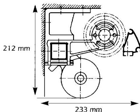
Elément de Fixation Mural ou plafond
