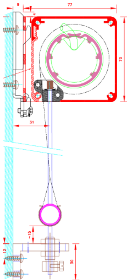
guidage câble
