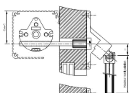
Treuil sortie 90°
