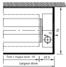
Treuil sortie dessous
