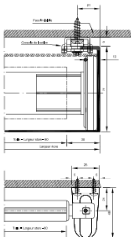
guidage câble
