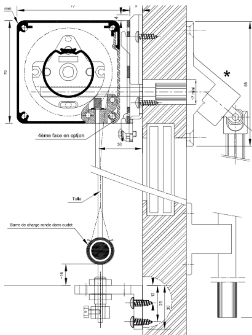
Treuil et manivelle renvoi intérieur 90°
