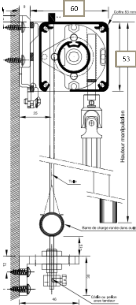
guidage câble
