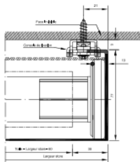
guidage câble
