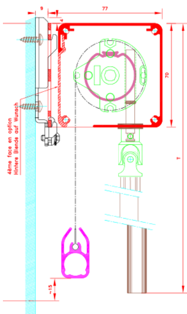
Treuil et manivelle sous coffre
